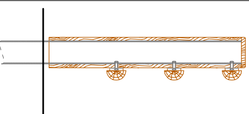
SEZIONE VERTICALE
